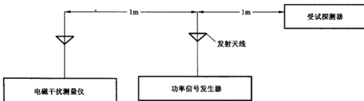
图 1 试验设备布置图
