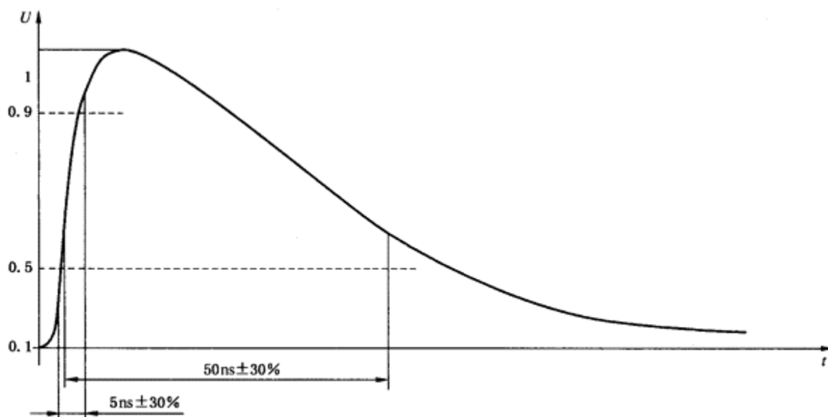
图 3 50 Ω 负载时单脉冲波形
