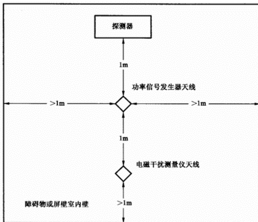
图 2 天线位置图
